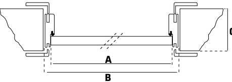
A - Door width | Largeur de la porte | Largura da porta B - Interspace | Largeur d'ouverture | Largura do vão C - Wall thickness | Épaisseur du mur | Espessura de parede
