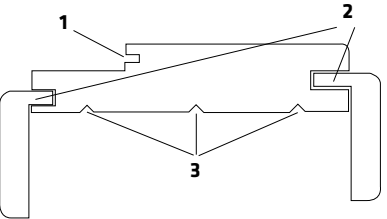
1 - Groove for rubber fixation | Fraiser pour le caoutchouc de montage | Rebaixe para fixação borracha 2 - Zone setting of the extensible casing | Zone de fixation de d'enveloppe extensible | Zona fixação da guarnição extensível 3 - Chase about to balance from wood | Rainure pour l'équilibre du bois | Ranhuras para equilíbrio da madeira
